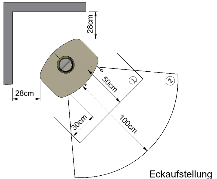
1...Feuerschutzplatte 2...Strahlungsbereich
