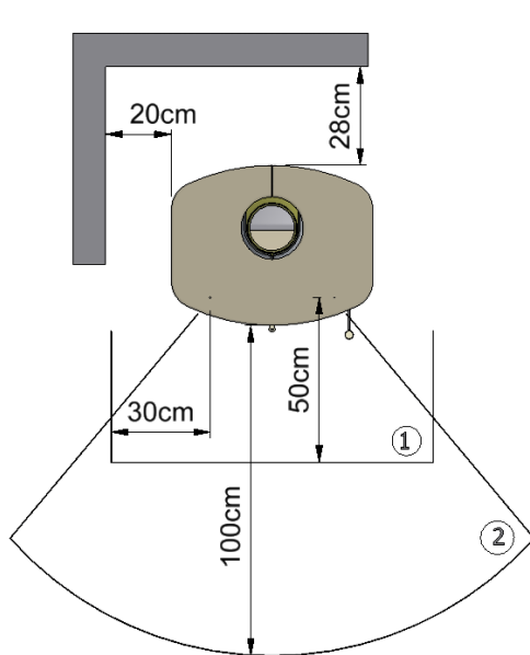
Wandaufstellung
