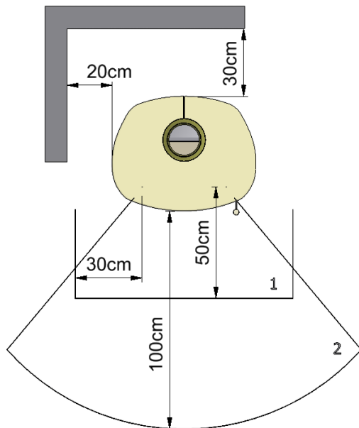
Wandaufstellung
