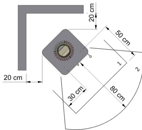
Eckaufstellung
