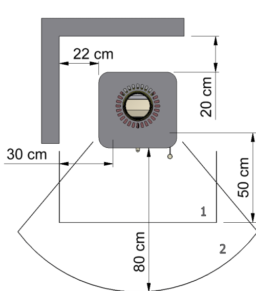
Wandaufstellung
