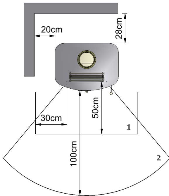
Wandaufstellung
