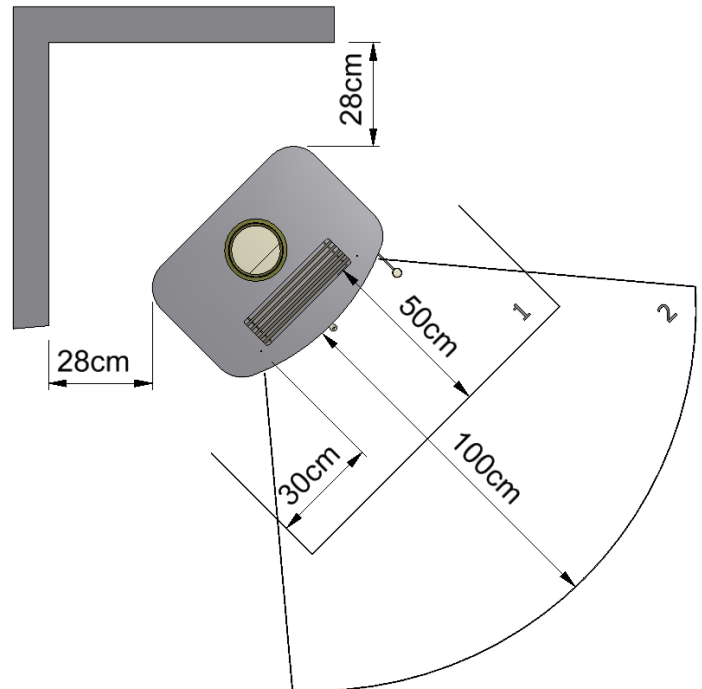
Eckaufstellung
