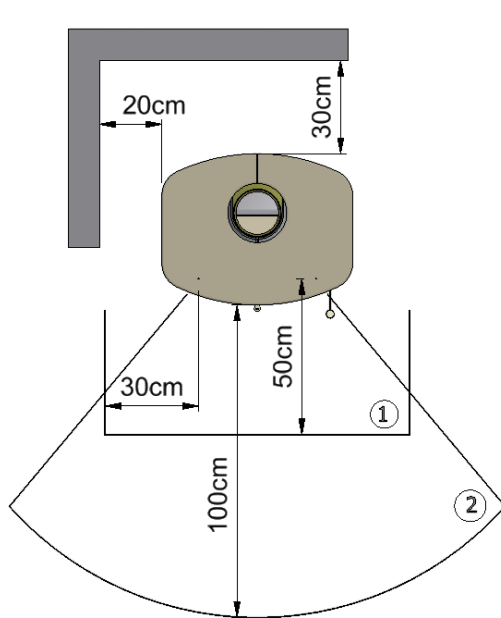
Wandaufstellung
