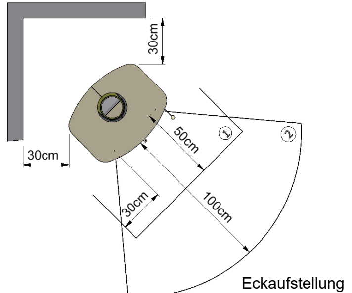
1...Feuerschutzplatte 2...Strahlungsbereich
