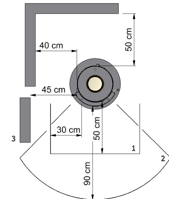
Wandaufstellung
