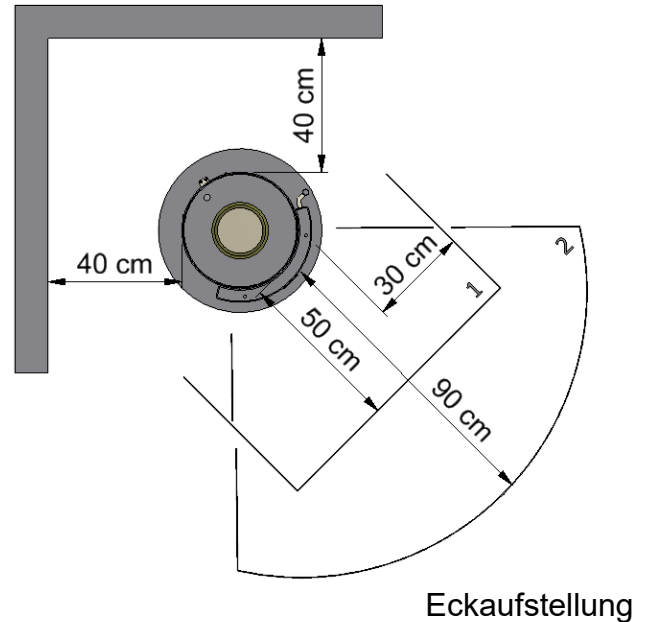
Eckaufstellung 1...Feuerschutzplatte 2...Strahlungsbereich
